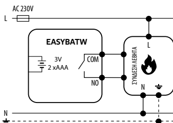
γ) Διάγραμμα σύνδεσης στην λωρίδα ελέγχου
