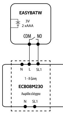
γ) Διάγραμμα σύνδεσης στην λωρίδα ελέγχου
